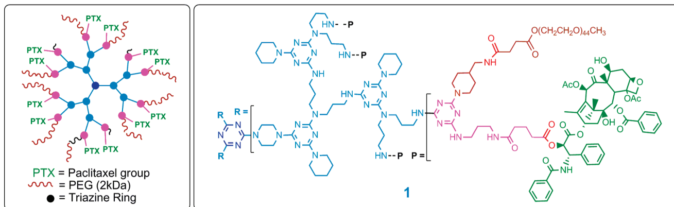
Chart 1. Dendrimer 1
